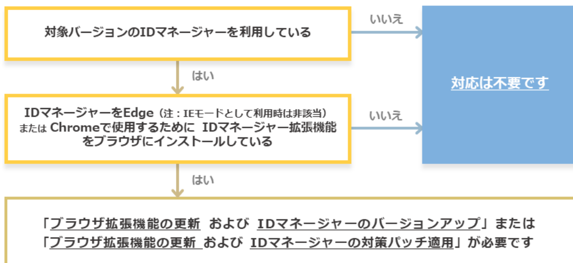
図 2 Manifest V2 サポート終了に伴う ID マネージャーの対応チャート
